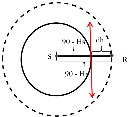
Bild 5. Astronomisk ortlinje.
