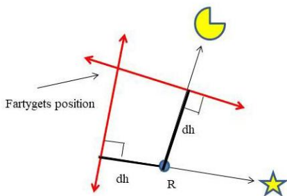
Bild 6. Sammanställda ortlinjer.
